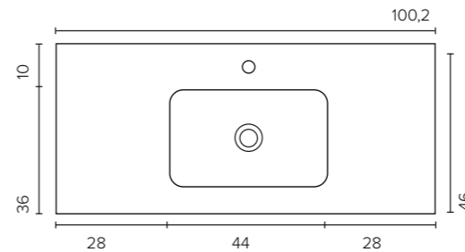
Sten (B x D x H) 100 x 46 x 2,5 cm | 0 - 1 hanehul
