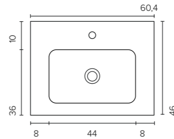
Sten (B x D x H) 60 x 46 x 2,5 cm | 0 - 1 hanehul
