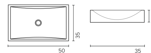
Top 5. Sten rektangulær uden hanehul
