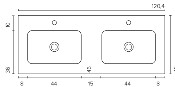
Sten (B x D x H) 120 x 46 x 2,5 cm | 0 - 2 hanehuller
